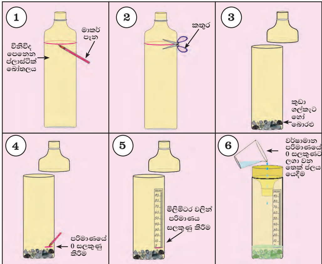
3.3.7 රූපය සරල වර්ෂාමානයක් සකස් කිරීමට උපදෙස්
