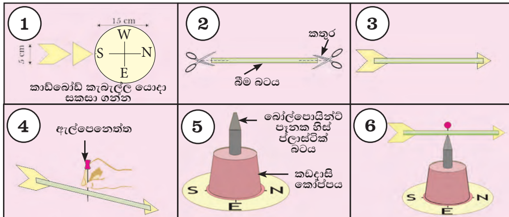
3.3.9 රූපය සරල සුළං දිශා දර්ශකයක් සකස් කිරීමට උපදෙස්
